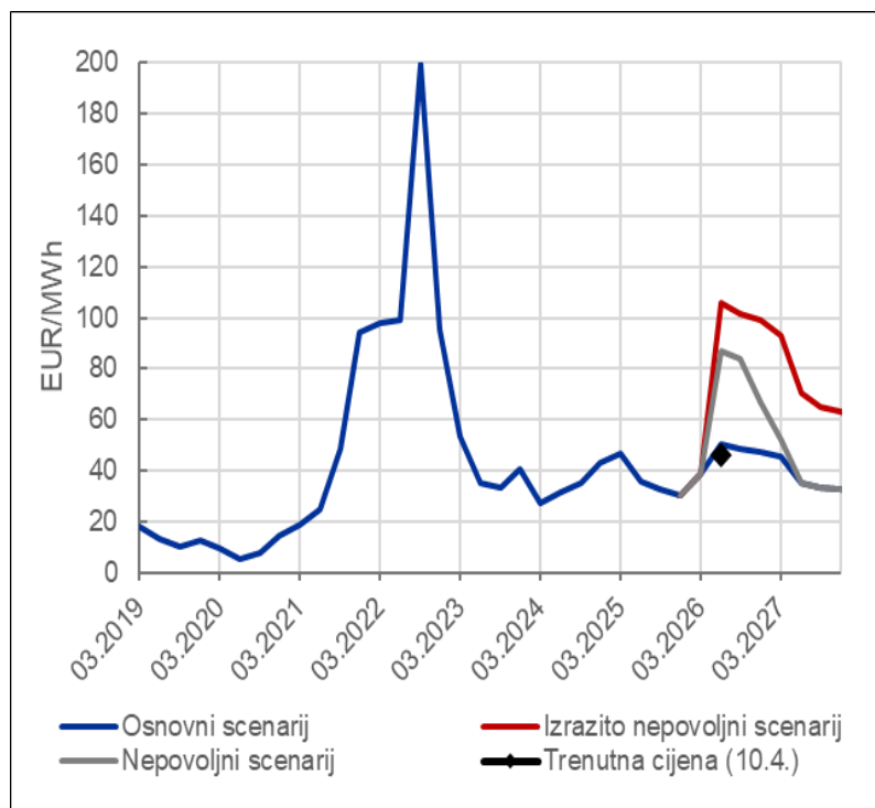
Plin
