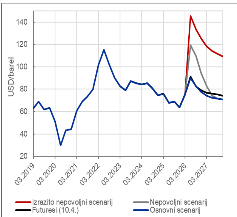
Nafta
